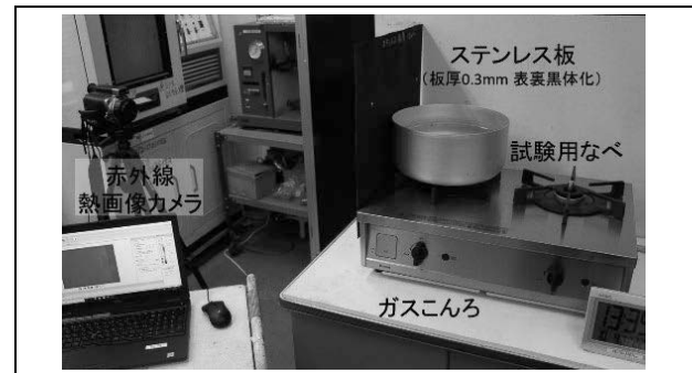
図5 ステンレス板防熱板受熱環境の実験状況
