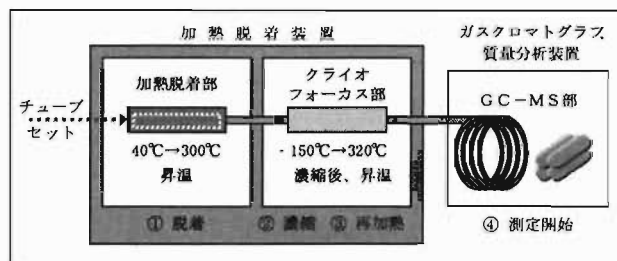
図1 装置構成
