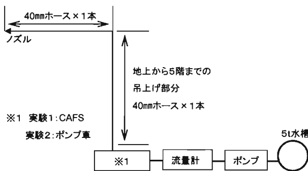
図4 放水体形図
