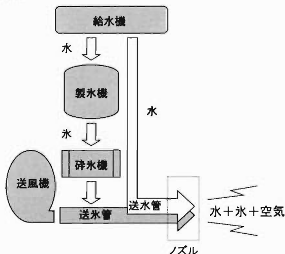
図1 基本構成図
