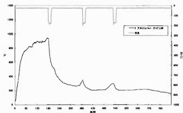
図10 実験8の温度と放水
