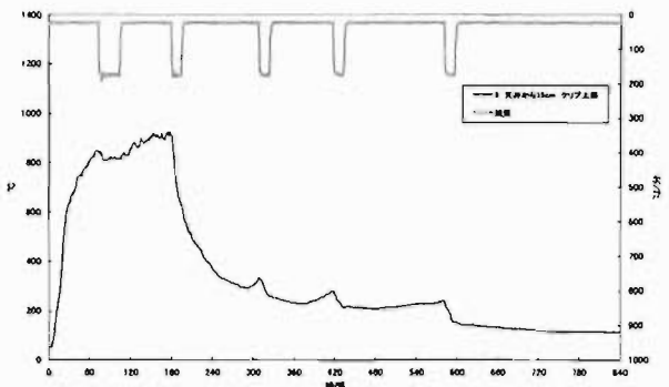
図9 実験7の温度と放水
