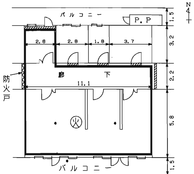
図2-1 火災室平面図
