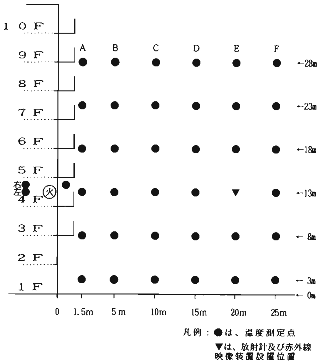
図3-2 実験の設定状況 (立面図)
