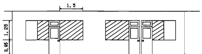
図2-2 火災室立面図
