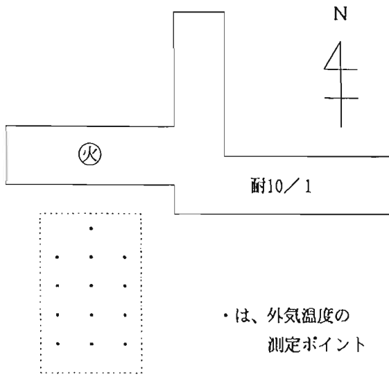
図1 実験建物の配置図
