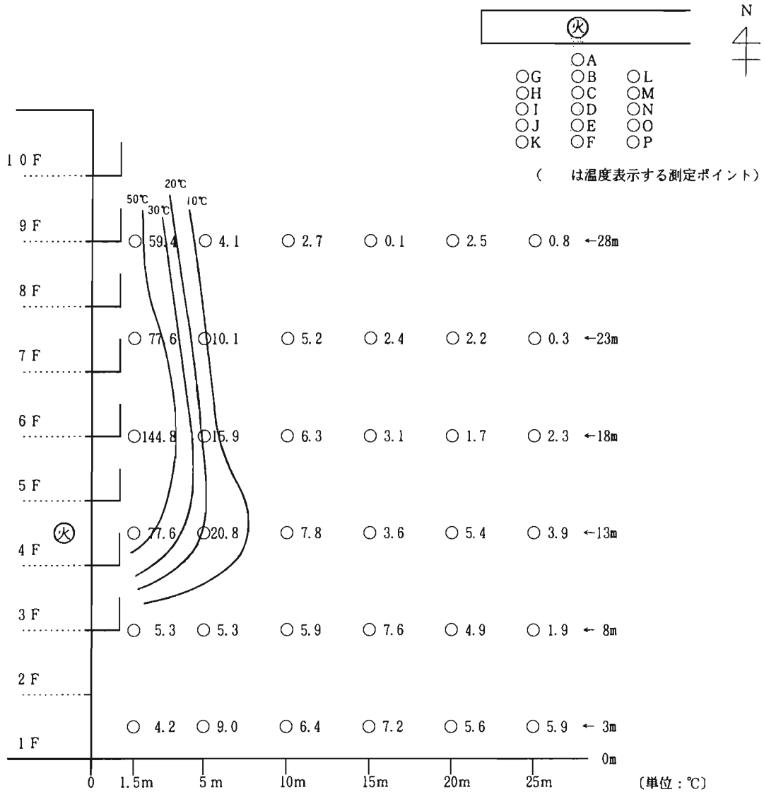
図6 点火後15分50秒における温度上昇値と推定等温線
