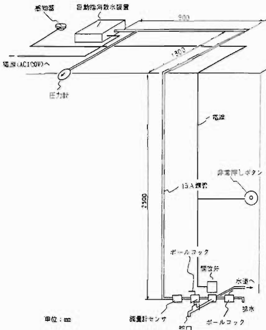
図4 散水装置概要図
