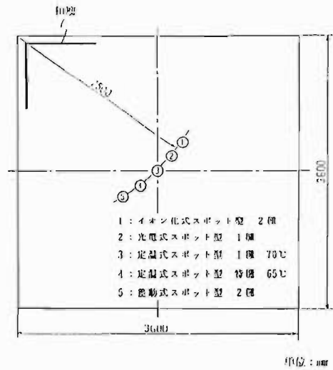
図6 感知器取付位置概要図
