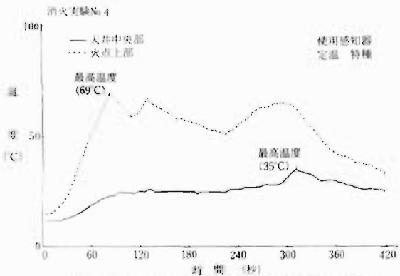
図16 ダンボール襖燃焼時の温度推移特性
