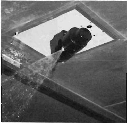
写真1 自動指向散水装置（試作1）
