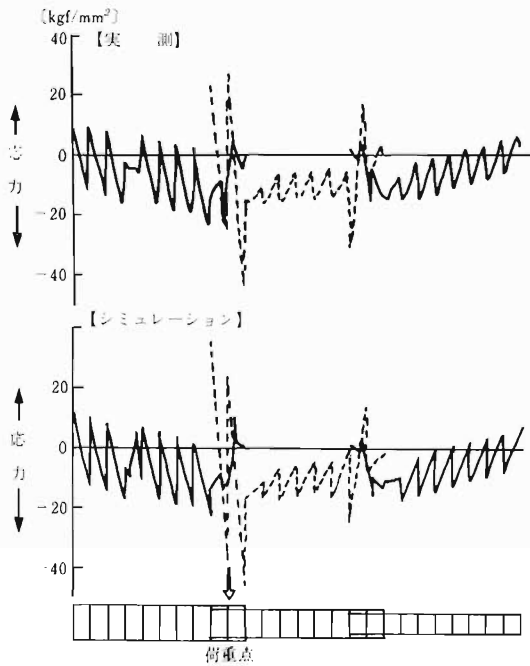
図4 応力分布 (水平全伸てい荷重80kg)
