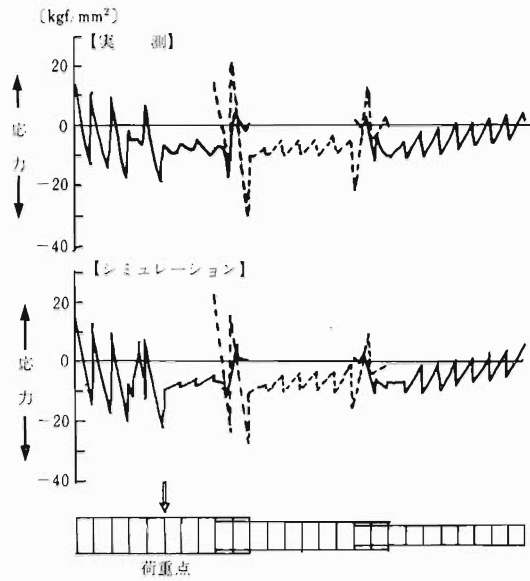
図3 応力分布 (水平全伸てい荷重80kg)
