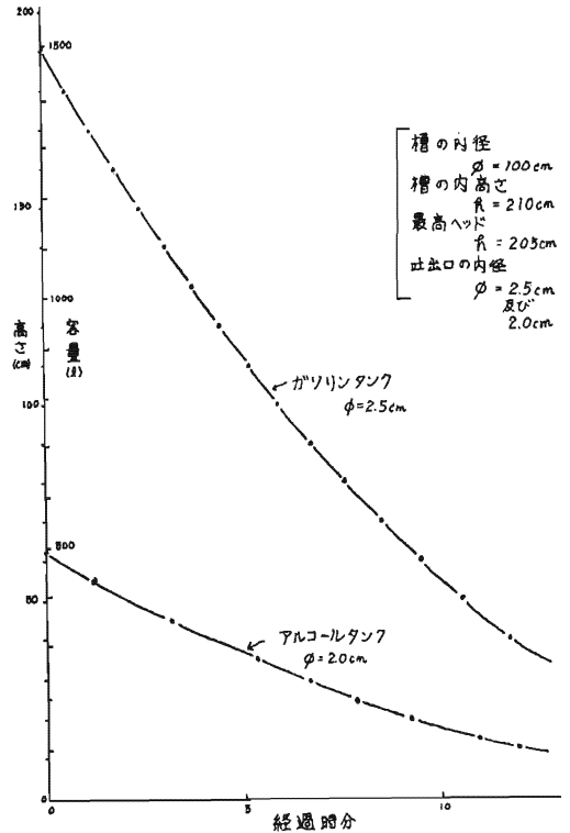
図4 各貯蔵タンクの流出速度実験結果
