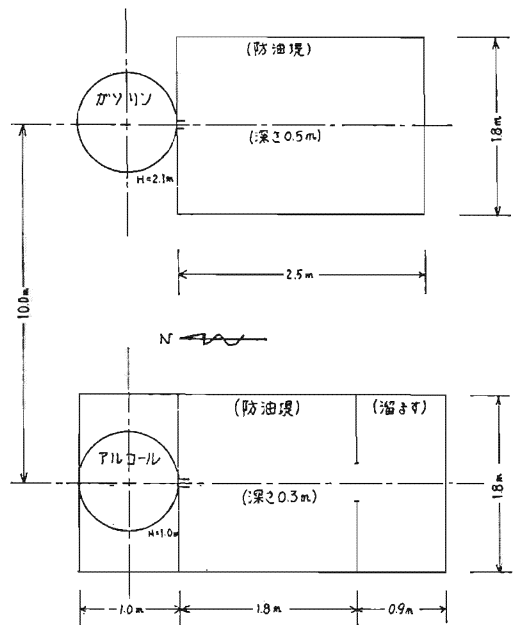
図1 貯蔵タンク及び防油堤の設定図
