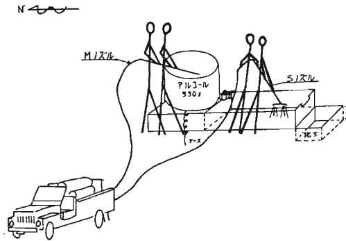
図3 アルコール処理状況図
