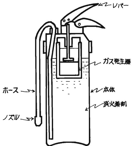
第1図 定圧式消火器概要図
