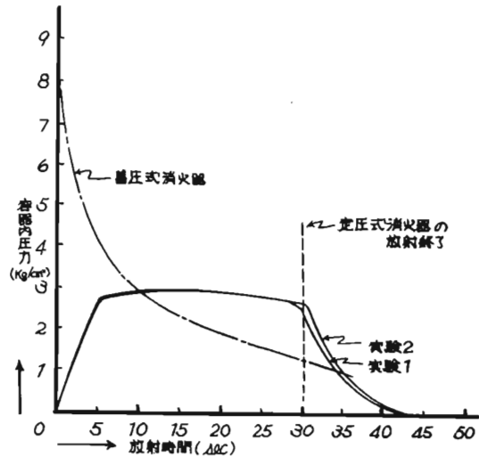
第3図 容器内圧力と放射時間との関係
