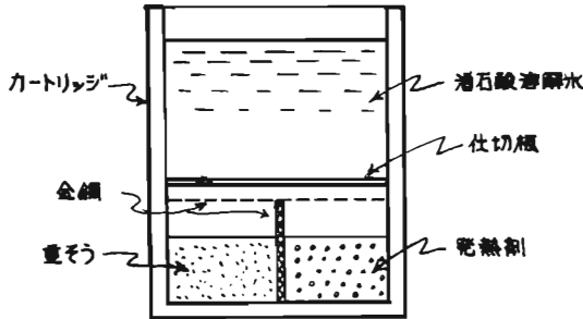
第2図 ガス発生器概要図
