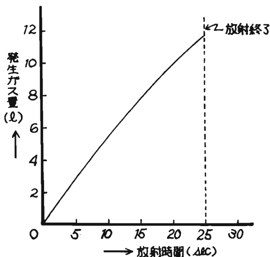
第4図 発生ガス量と放射時間
