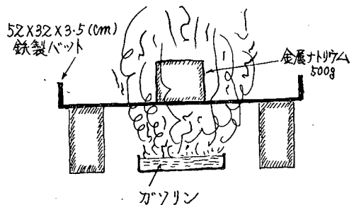
第2図 金属ナトリウムの点火方法
