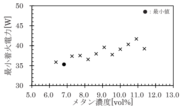
図 18 メタン濃度に対する最小着火電力
