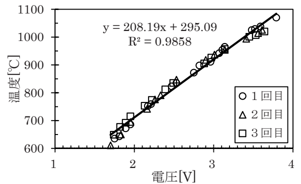
図10 電熱線温度測定実験結果の電圧 - 温度関係図
