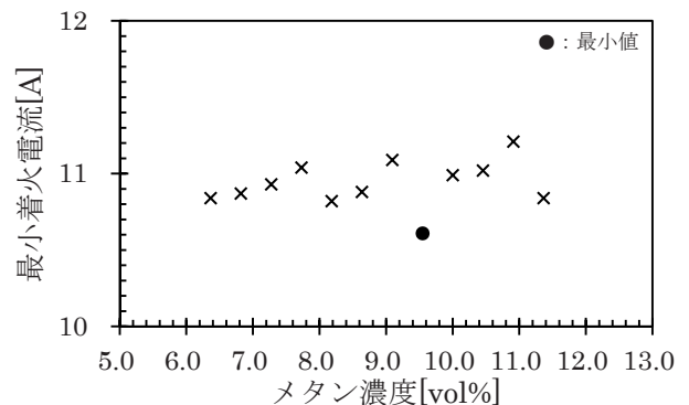
図 17 メタン濃度に対する最小着火電流
