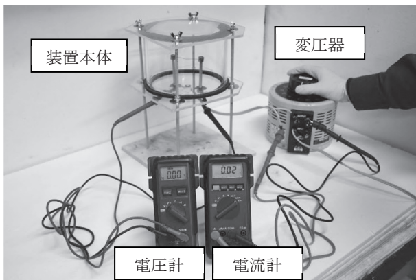
図3 電熱線着火実験装置全体図
