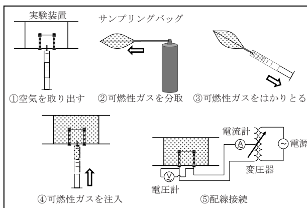
図7 可燃性ガス混合気の調製手順
