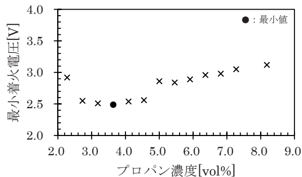
図13 プロパン濃度に対する最小着火電圧
