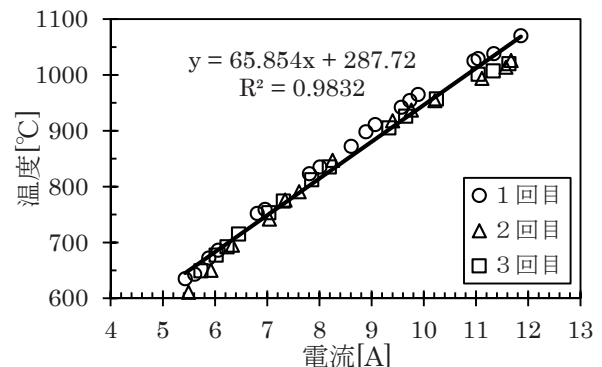
図11 電熱線温度測定実験結果の電流 - 温度関係図
