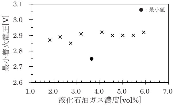
図 19 液化石油ガス濃度に対する最小着火電圧
