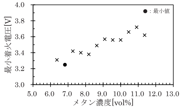
図 16 メタン濃度に対する最小着火電圧
