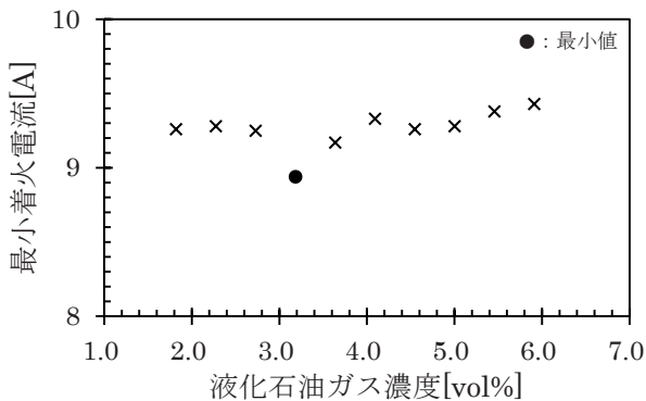
図 20 液化石油ガス濃度に対する最小着火電流
