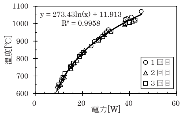
図12 電熱線温度測定実験結果の電力 - 温度関係図
