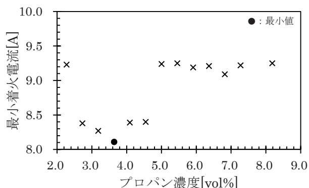
図14 プロパン濃度に対する最小着火電流
