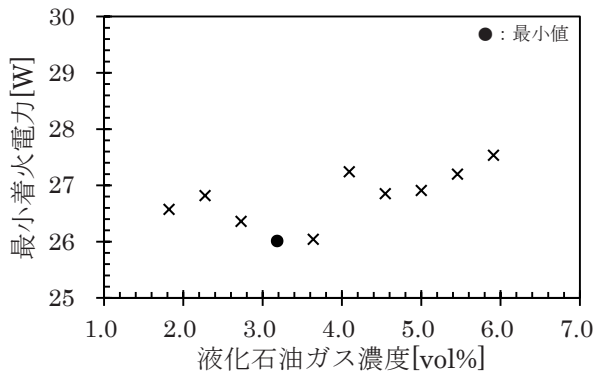
図 21 液化石油ガス濃度に対する最小着火電力
