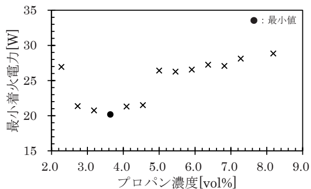
図15 プロパン濃度に対する最小着火電力
