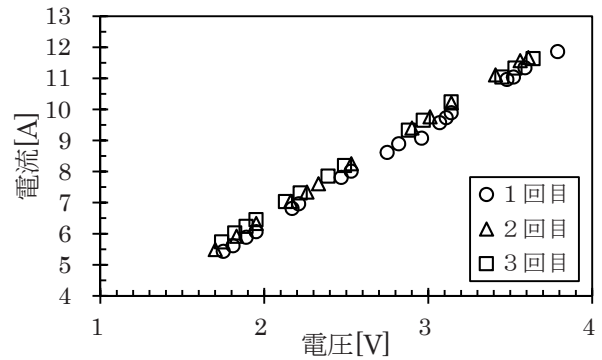
図9 電熱線温度測定実験結果の電圧 - 電流関係図
