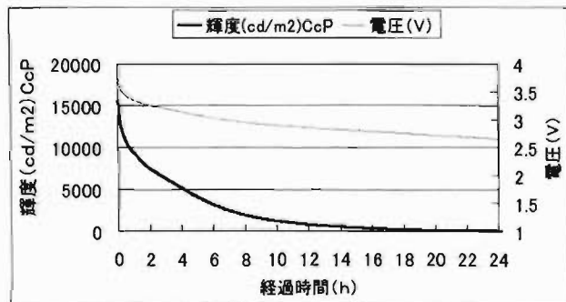
図4 LED 輝度と電圧の時間変化
