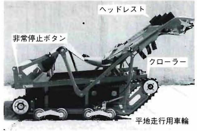
写真2 救出用台車の外観（側面）
