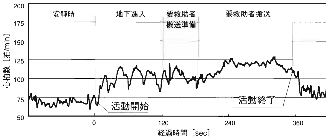
図4 心拍数の時系列変化 (台車による救出時) (隊員 F)
