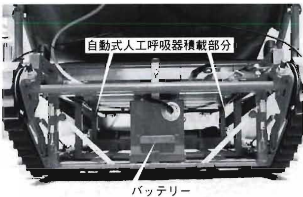
写真3 自動式人工呼吸器積載部分
