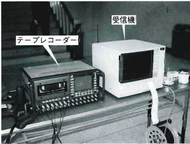
写真7 受信機及びデータレコーダ設置状況
