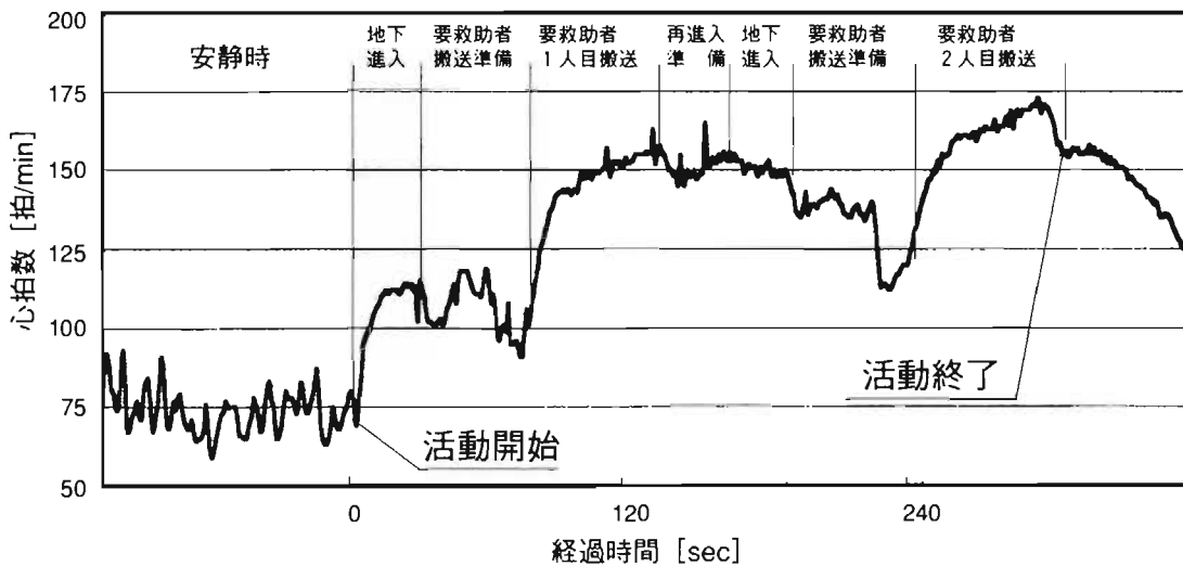
図5 心拍数の時系列変化 (平担架による救出時) (隊員 F)
