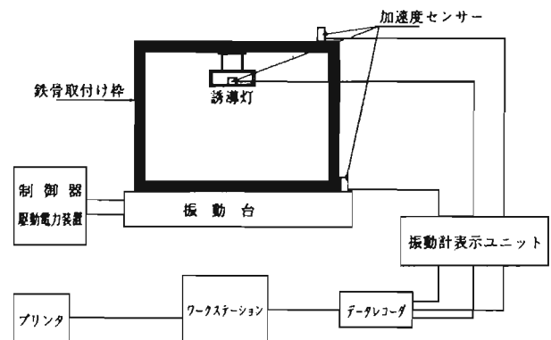
図24 測定系統図
