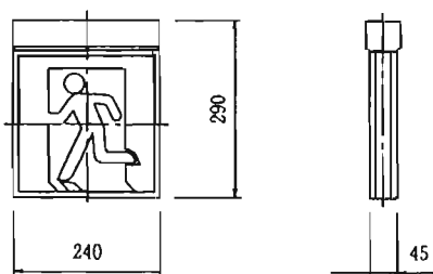
図8 高輝度誘導灯 (A社製)
