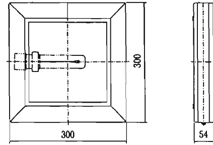
図9 高輝度誘導灯 (C社製)
