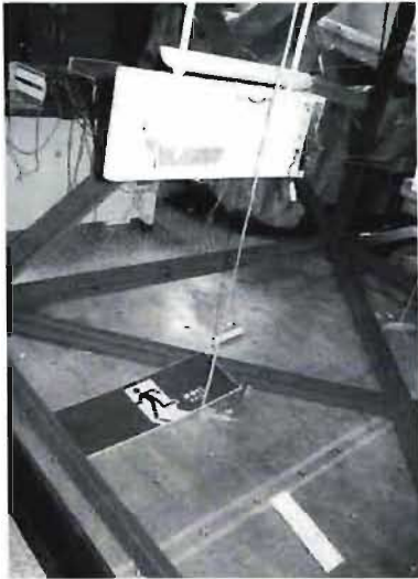
写真4 パネルとバッテリーが落下した状況
