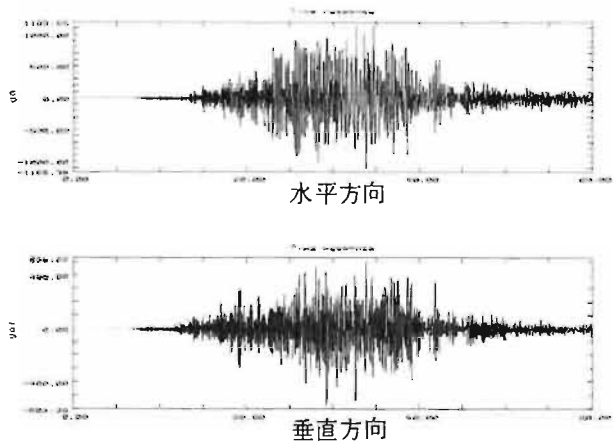
図3 ラック中段の応答加速度波形
