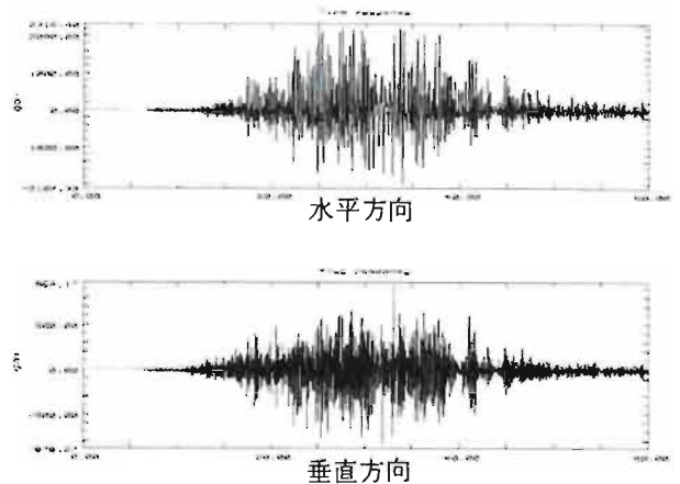
図6 実験3のときプリンタの応答加速度波形
