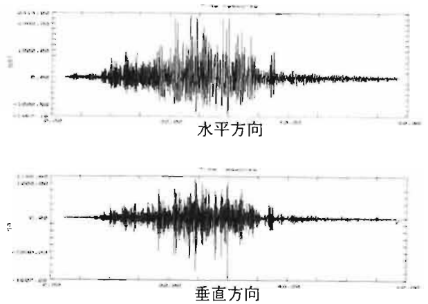
図5 実験2のときプリンタの応答加速度波形
