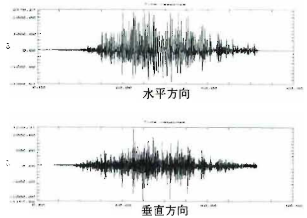
図4 実験1のときプリンタの応答加速度波形
