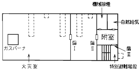
図1-2 火災階平面図
