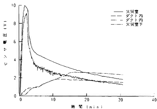
図12 火災室及びその上下室に通じるダクト内の燃焼生成ガス濃度変化(CASE-5)
