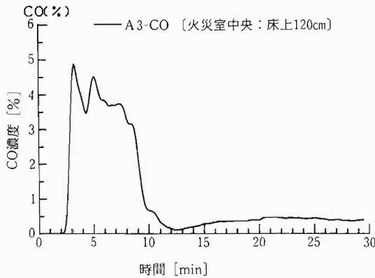
図8 火災室内のCO濃度変化 (扉開放)
