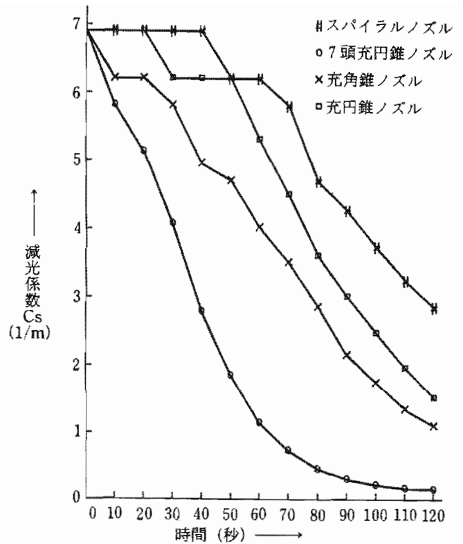
図6 各種ノズルの消煙効果(ノズル圧力20kg/cm 2 )
