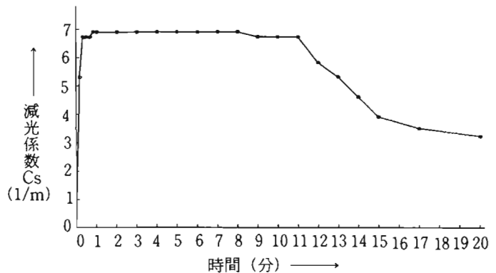
図4 発煙筒の煙濃度(自然減衰状況)
