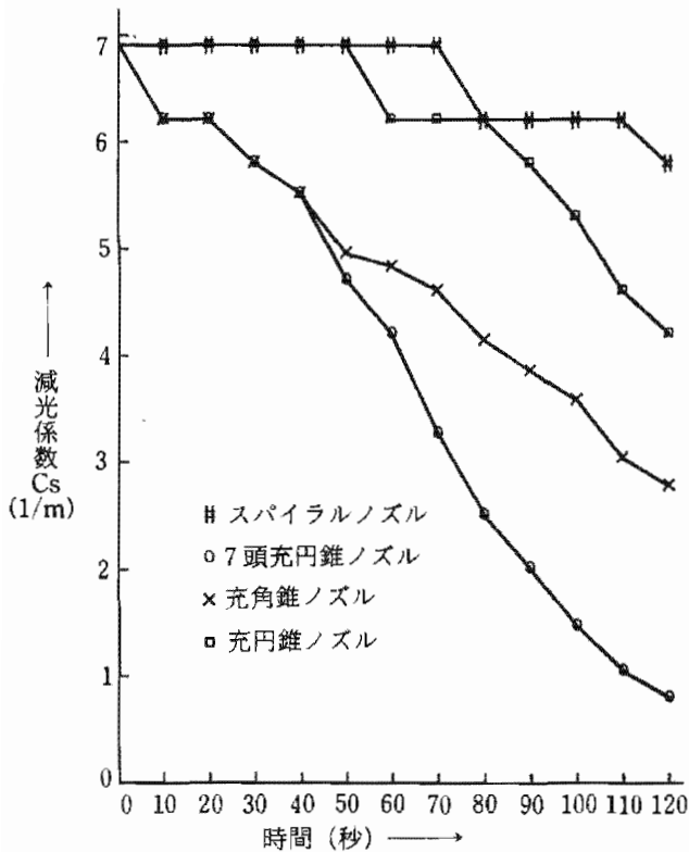
図5 各種ノズルの消煙効果(ノズル圧力10kg/cm 2 )
