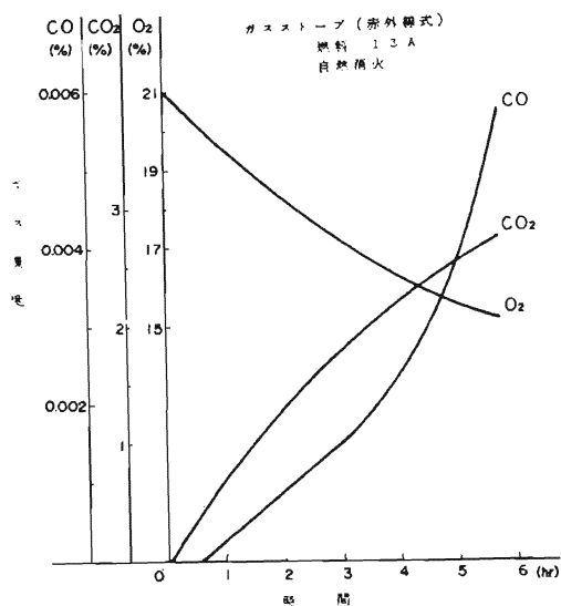
図3 ガスストーブ (赤外線式) のガス濃度変化 なお、6B用器具については前回 (所報第15号) 掲載済みである。
