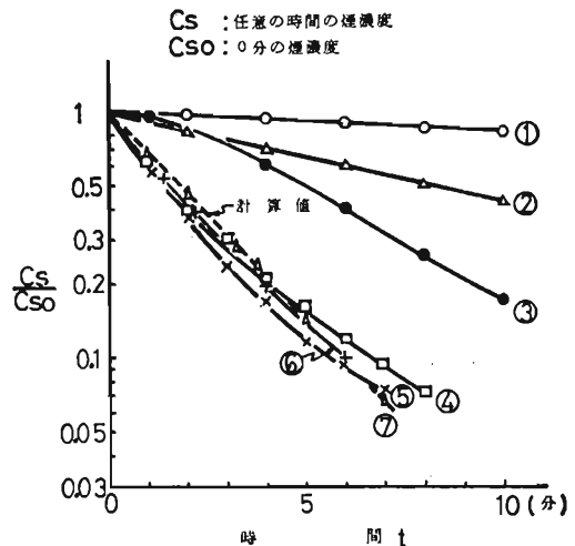
図3 消煙、排煙性能の比較
