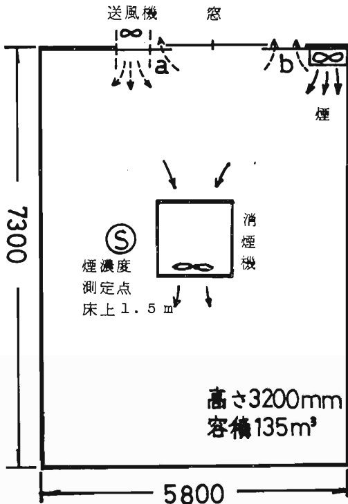
図1 消防訓練塔消煙実験室
