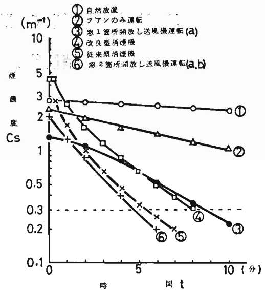
図3 消煙、排煙性能の比較
