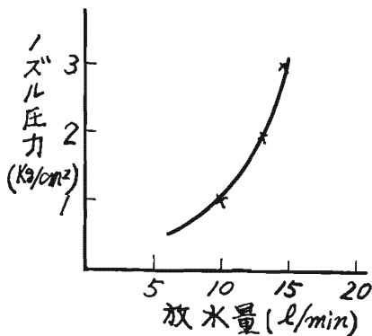
第3図 放水曲線 (展開角度40°)
