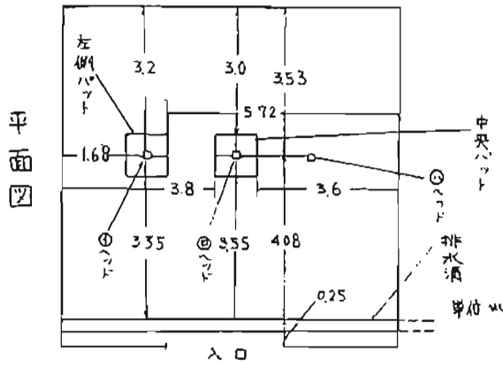
第5図 感熱装置 (スプリンクラーヘッド) のハット及びバット配設図
