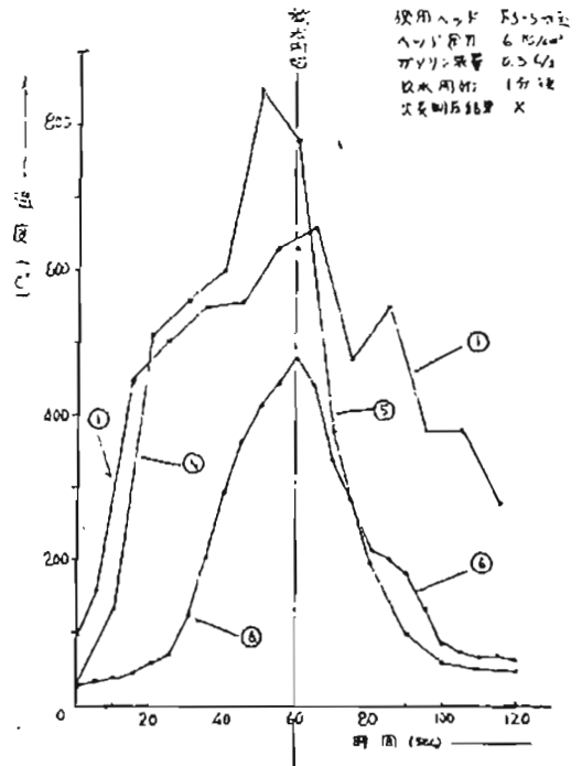
第12表 着火より放水開始までの時間と温度
