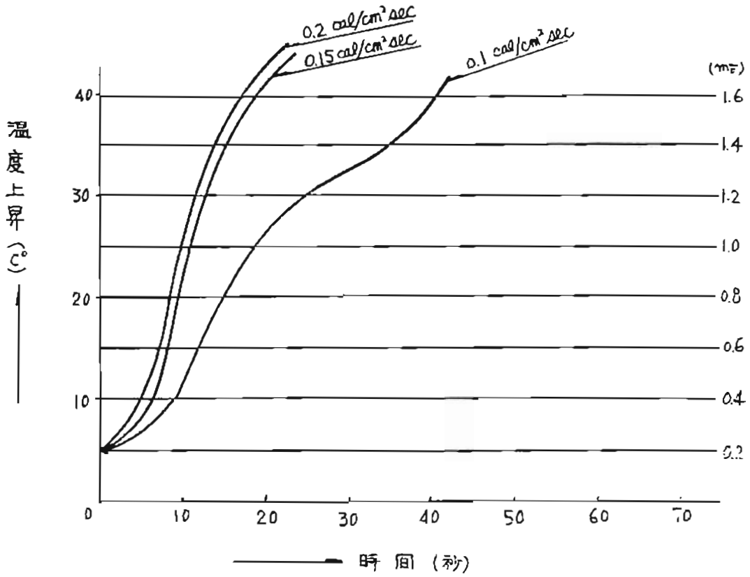
第A-2図 三又刺子放射加熱総合曲線
