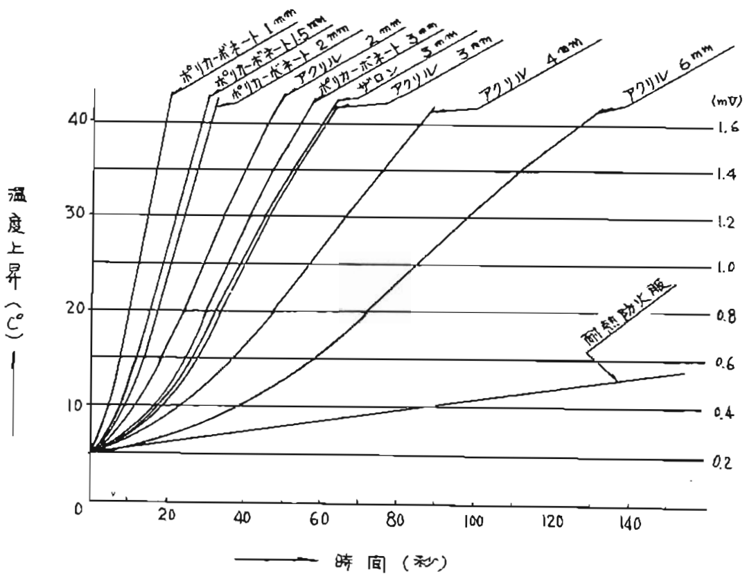
第B-1図 0.1cal/cm².sec 合成樹脂総合曲線
