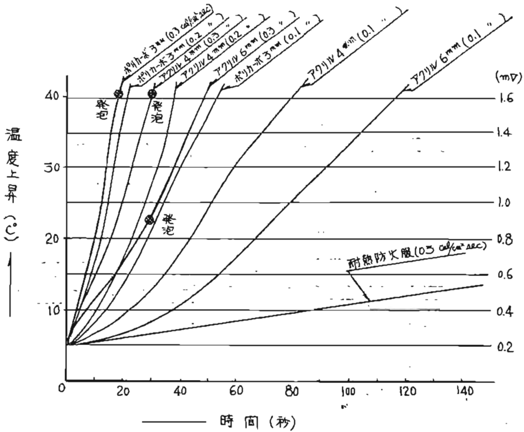
第B-2図 各種放射加熱試験による合成樹脂総合曲線
