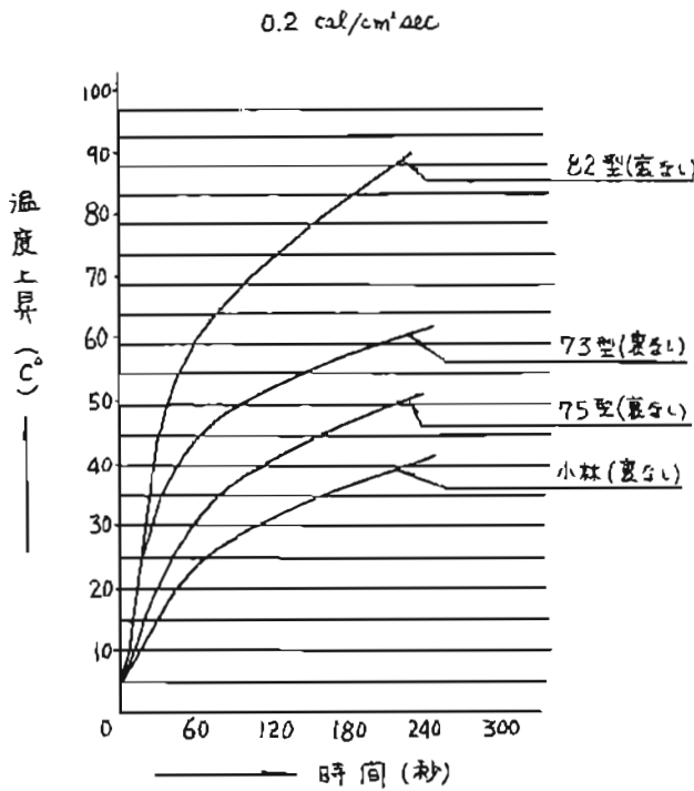
第D-1図 耐熱服裏面温度上昇総合曲線
