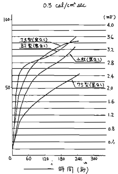
耐熱服裏面温度上昇総合曲線
