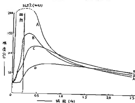
第5図 実験2の14秒加熱曲線
