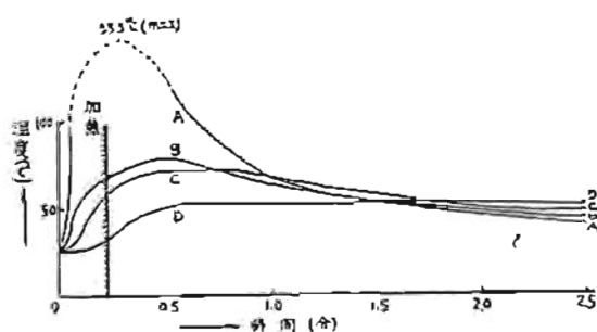
第5図 実験2の14秒加熱曲線
