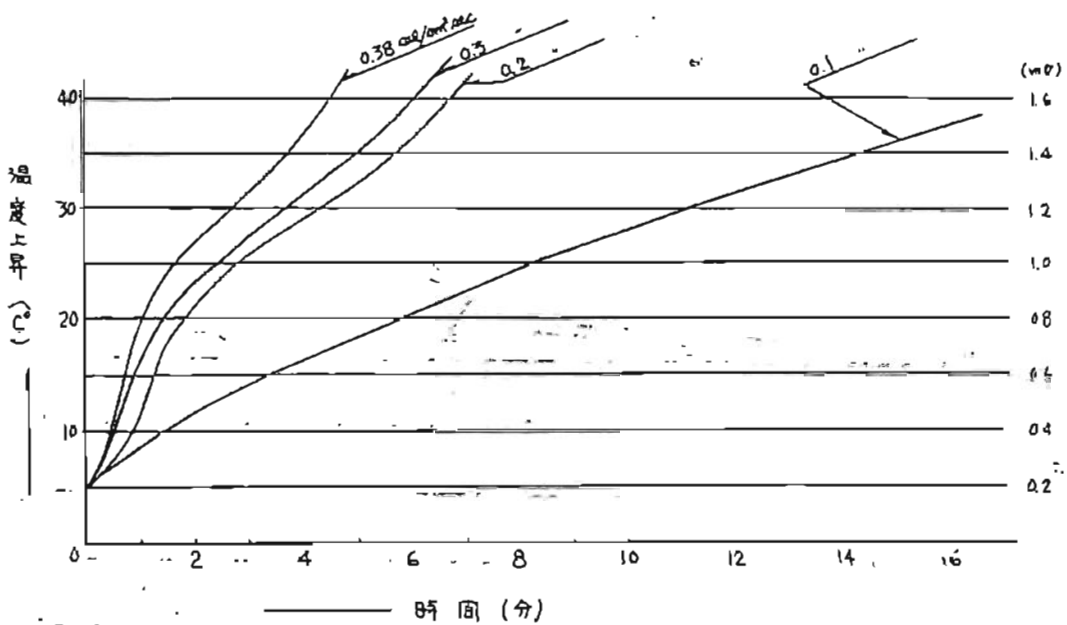
第A-1図 耐熱防火服小林刺子製総合曲線
