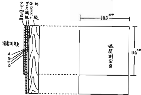
第2図 温度測定点
